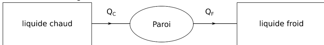
Transferts thermiques à travers la paroi d'un échangeur
