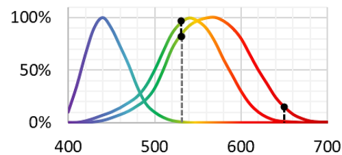
stimulus dû à une addition de lumières rouge et verte
