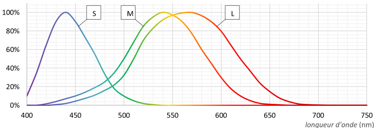
sensibilités des trois types de cônes (en pourcentage de leur valeur maximale)
