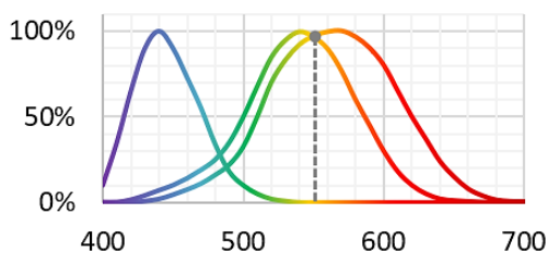
stimulus dû à une lumière monochromatique jaune
