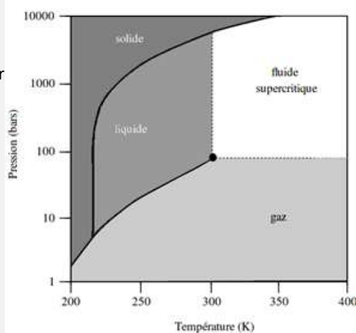
Diagramme de phases du dioxyde de carbone
